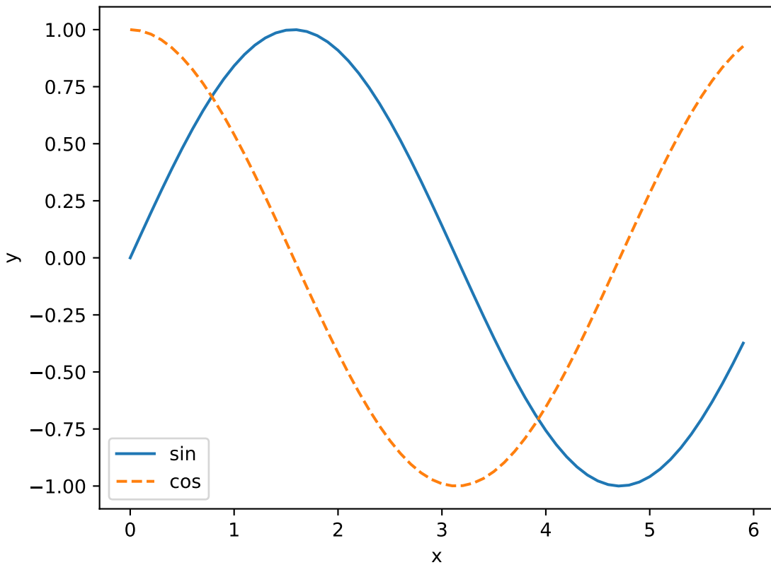
sin & cos
